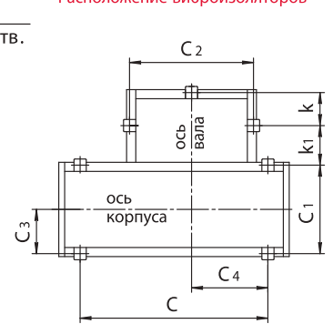
Расположение виброизоляторов
